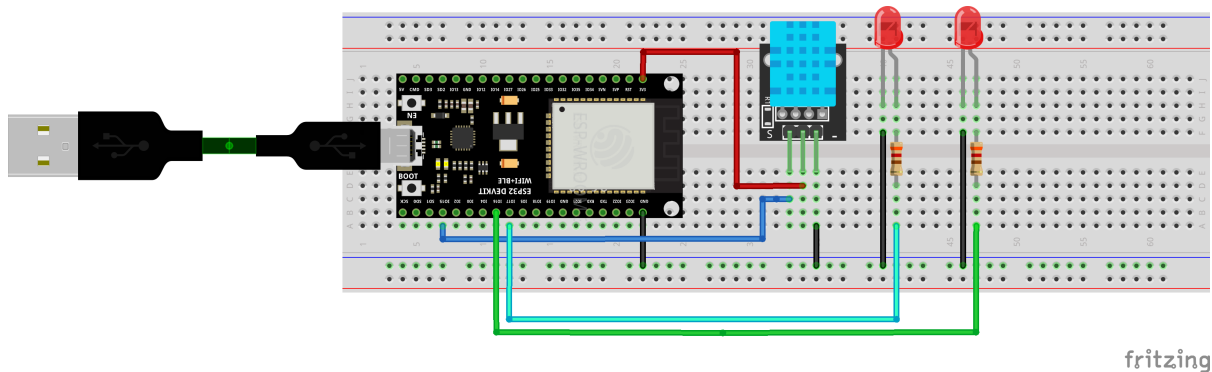
Figura 8.1: Diagrama de circuito de la casa inteligente
