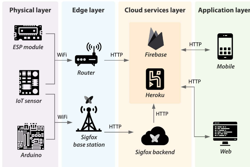
Figura 6.1: Arquitectura general de sistemas IoT utilizados en proyectos académicos [2]
