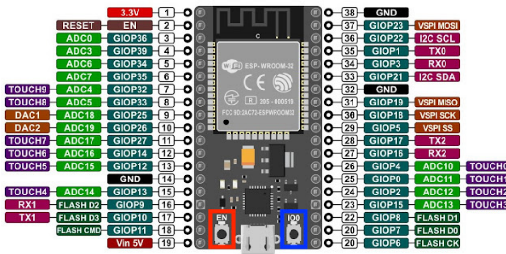
Figura 8.4: Botones de la ESP32
